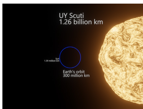
El tamaño de UY Scuti comparado con la órbita de la Tierra y el Sol (apenas visible).
